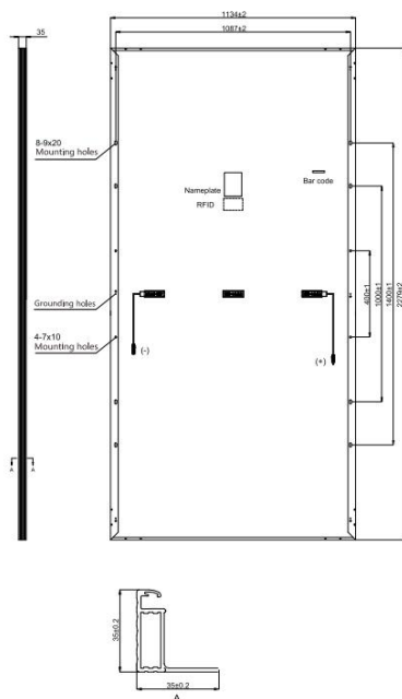
Dimensiones del módulo fotovoltaico
